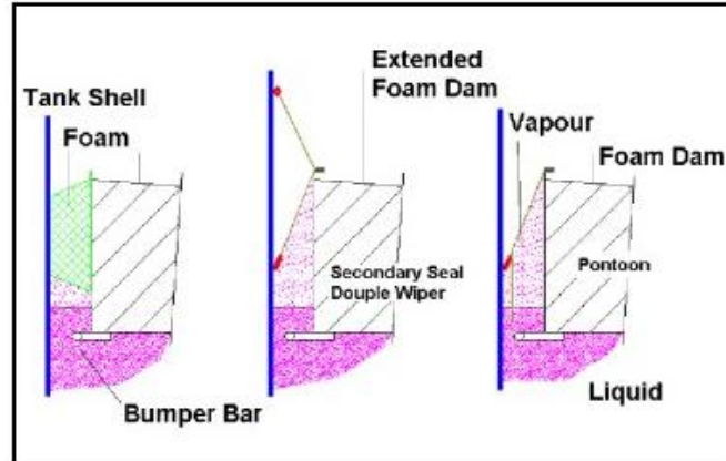
Şekil 4.2: Buhar montajlı contalar (tipik)
