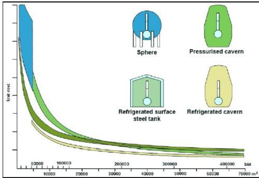
Unit Cost: Birim maliyet Sphere: Küre Pressurized Cavern: Basıncılı Çukur Refrigerated surface steel tank: Soğutulmuş yüzey çelik tankı Refrigerated cavern: Soğutulmuş çukur
