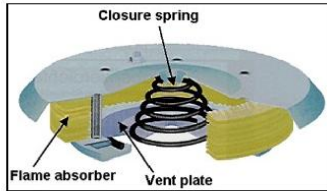
Şekil 4.21: Boşaltım menfezi örneği (patentli tasarım)
