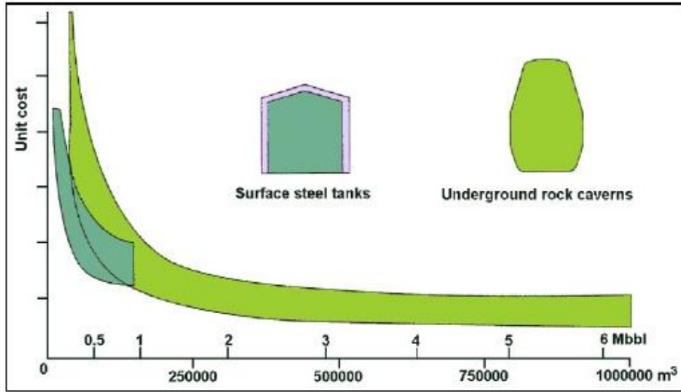
Unit cost: Birim maliyet Surface Steel tanks: Yüzey çelik tankları Underground rock caverns: Yer altı kayaç çukurları
